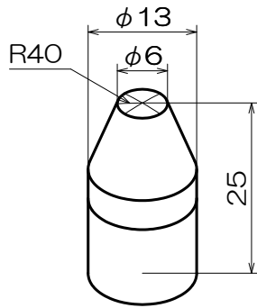
H-433 CF形（円錐形）φ13 10個入
