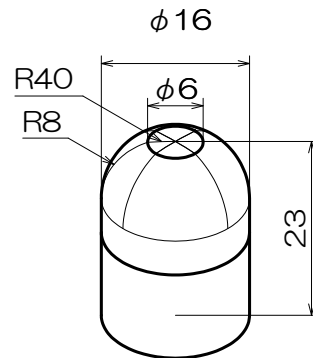
H-464 DR形（ドーナツ形）φ16-6 10個入
