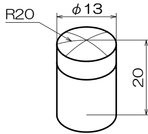
H-481 R20形（ラッパ形）φ13 10個入
