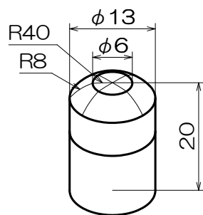
H-434 DR形（ドーナツ形）φ13 10個入
