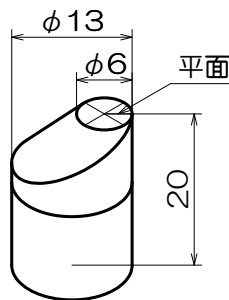
H-436 EF形（偏心形）φ13 10個入
