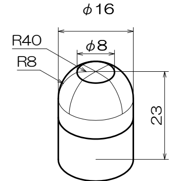
H-474 DR形（ドーナツ形）φ16-8 10個入
