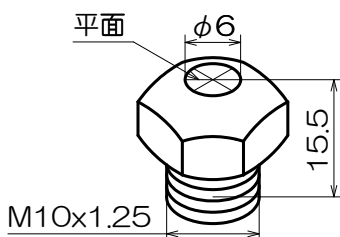
H-438 ベースチップφ6 10個入
