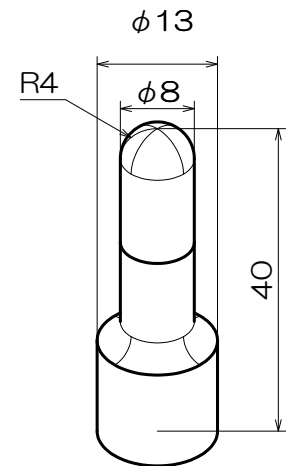
H-439 SD形（ステップドーナツ形）φ13 3個入
