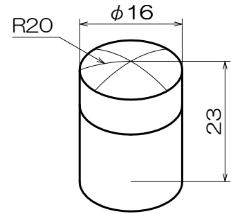
H-486 R20形（ラッパ形）φ16 10個入
